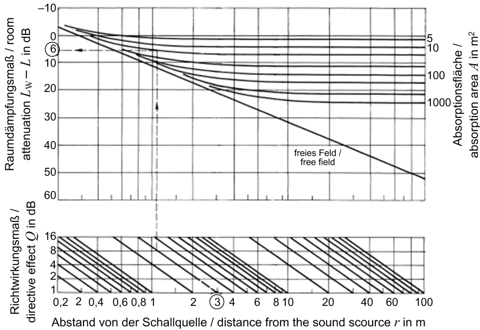
Bild 17. Raumdämpfung in Abhängigkeit von der äquivalenten Absorptionsfläche, vom Abstand von der Schallquelle und von der Richtungscharakteristik der Schallquelle
